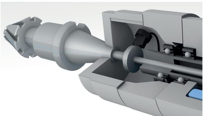
Détermination de la position d'une pince de serrage dans une broche porte-outil de machine avec un système de mesure de position inductif
