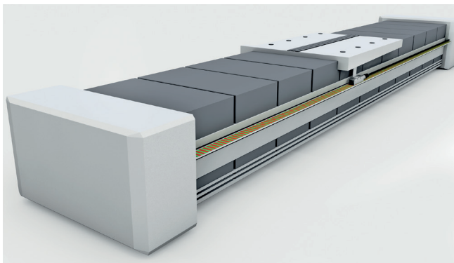
Signalisation en retour de la position de chariot actuelle avec un système de mesure de déplacement à codage magnétique linéaire
