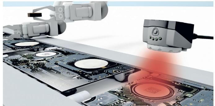
Identification de cartes électroniques au moyen de codes 2D à marquage direct à l'aide d'un lecteur de codes stationnaire
